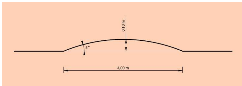
Figura 10. Esquema d'una esquena d'ase.
