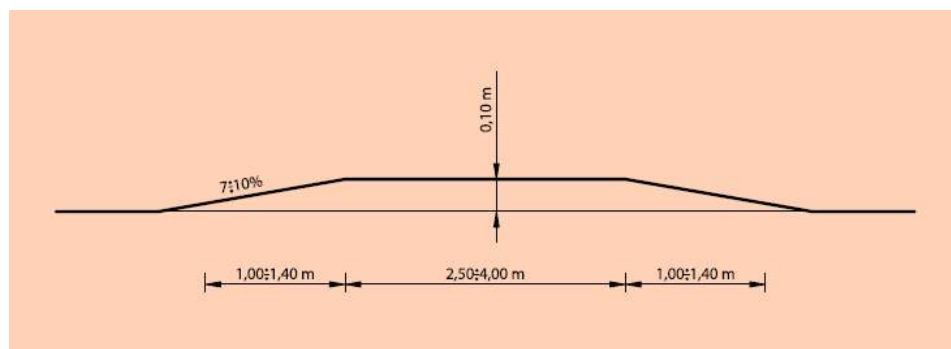
Figura 7. Esquema d'un pas de vianants de ressalt.
